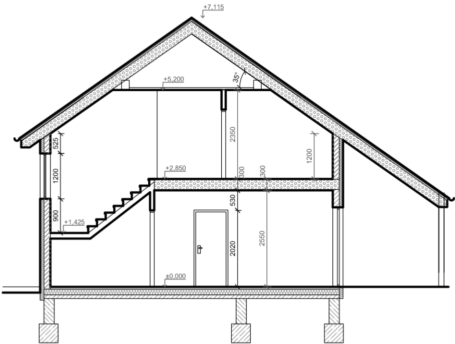
ŘEZ A-A
