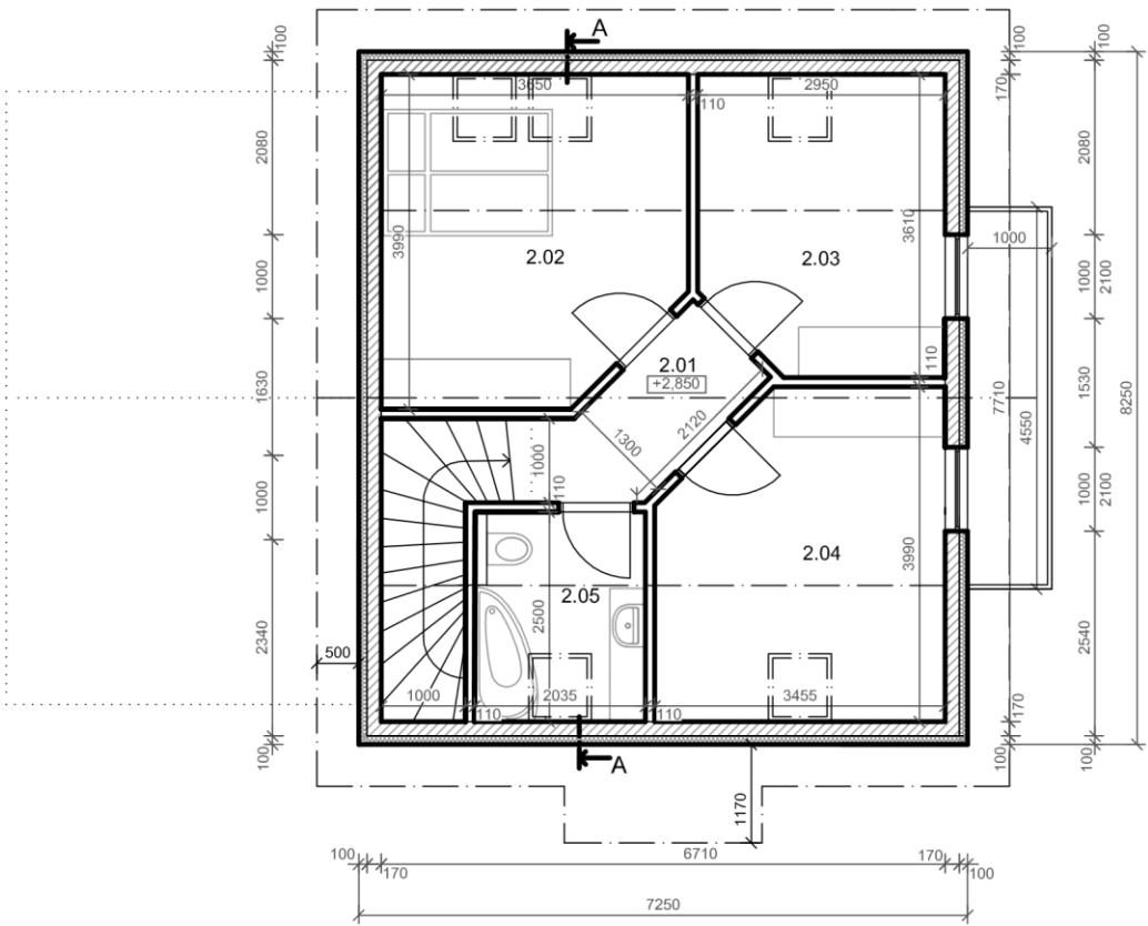
PŮDORYS 2. NP
