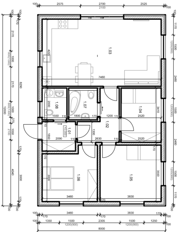
PŮDORYS 1. NP
